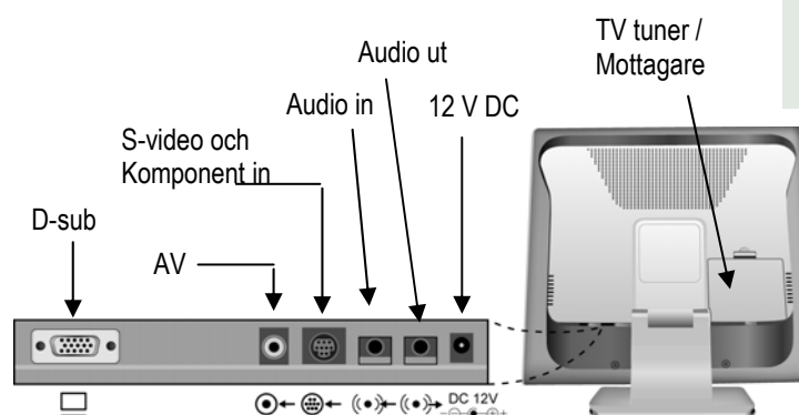
Figur 2. Multimediamonitor bakifrån.
